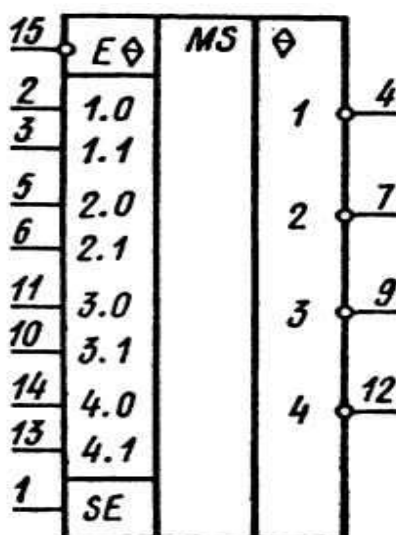
Условное графическое обозначение КР1533КП11А, КФ1533КП11А, ЭКФ1533КП11А
